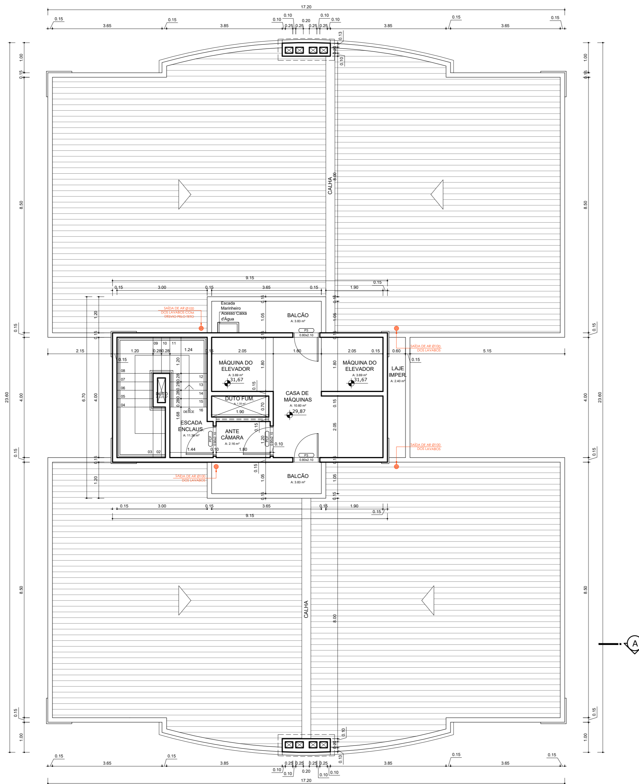
PLANTA BAIXA PAVTO CASA DE MÁQUINAS - TORRE 01/ 02/ 07/ 08/ 09 ÁREA DO PAVTO: 48,82 m²
